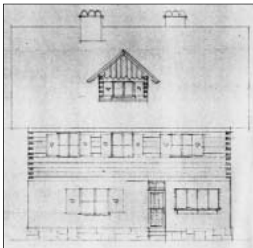
Plán lesníckeho domku - poľovníckej chaty Leopolda Haupt-Stummera z 21.8.1937
